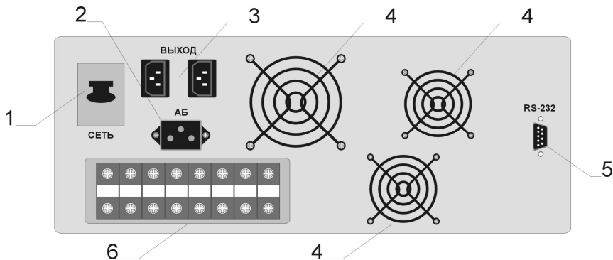
Рис. 2 Внешний вид задней панели ИБП:
