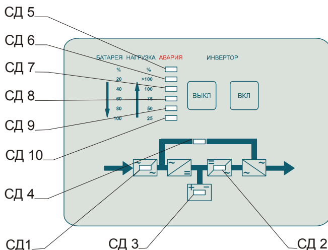
Рис. 1 Передняя панель блока ИБП
