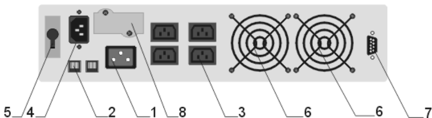
б) ДПК-1/1-2-220-Т, ДПК-1/1-3-220-Т
